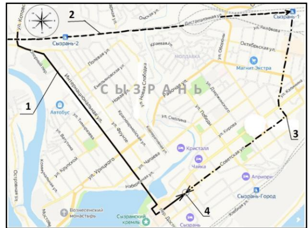
Рисунок 1. – Карта-схема перемещений О. Бендера и И.М. Воробьянинова по г. Старгороду, примененная к г. Сызрани
